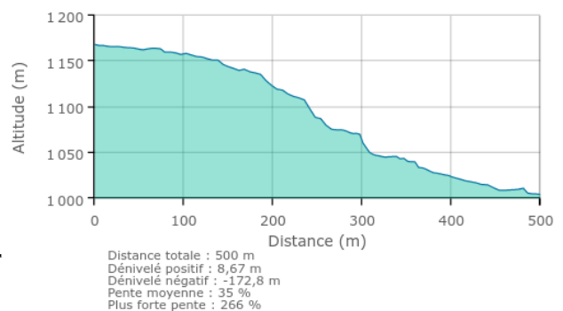
PROFIL ALTIMÉTRIQUE
